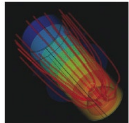
Simulación numérica de superficies térmicas y líneas de iso-concentración en un pellet.
